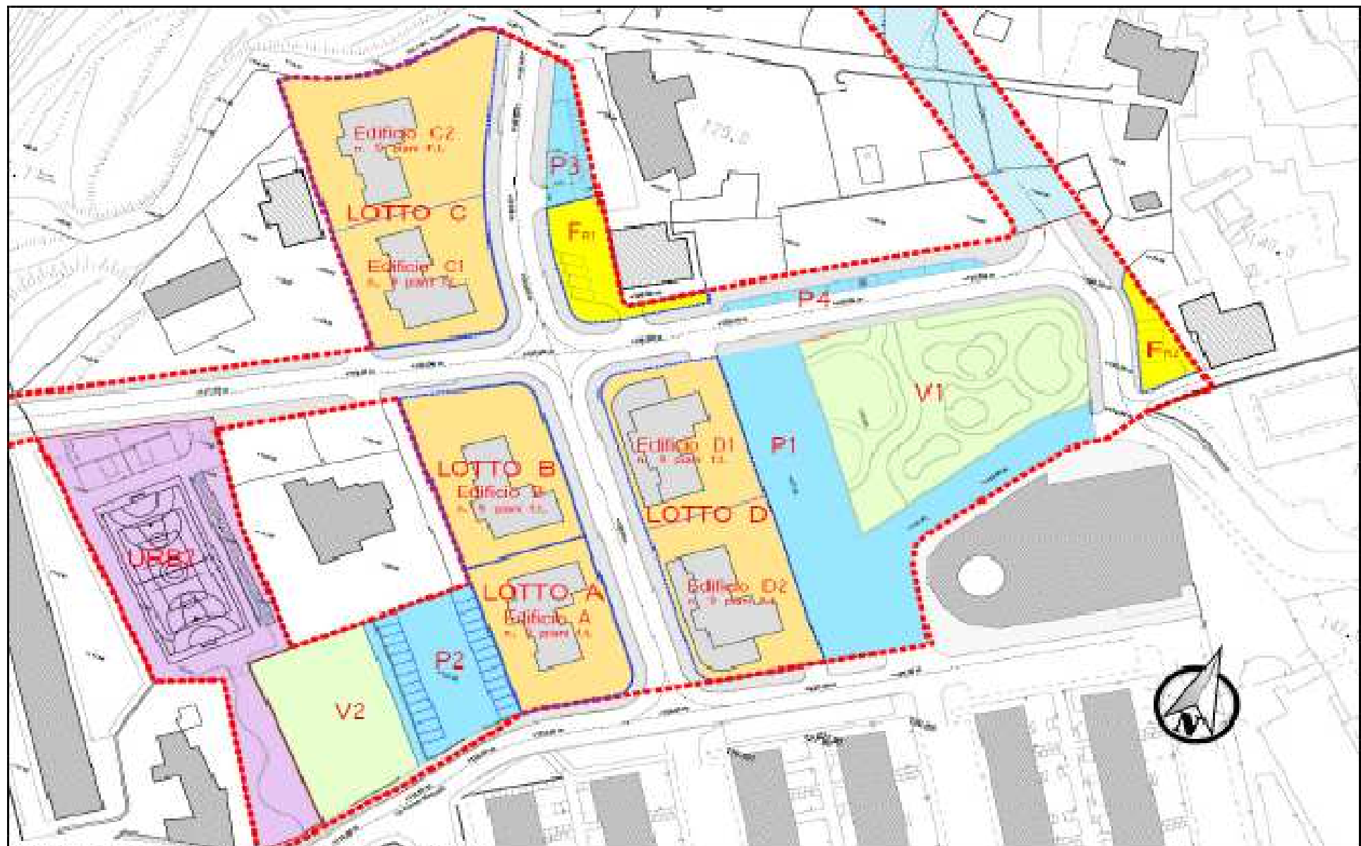
STRALCIO BOZZA ZONIZZAZIONE PUA
